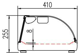
DOORSNEDE BCS
