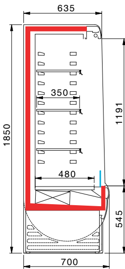
DOORSNEDE VENERE
