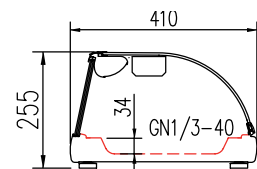
DOORSNEDE BCCS
