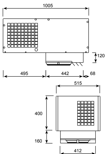
MAATSCHETS 1
