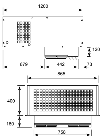
MAATSCHETS 2
