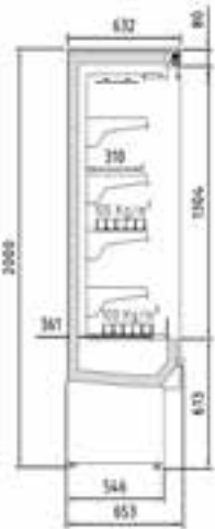
DOORSNEDE CDS
